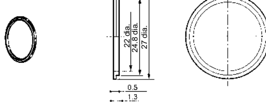
25-dia. Ring A22Z-R25
